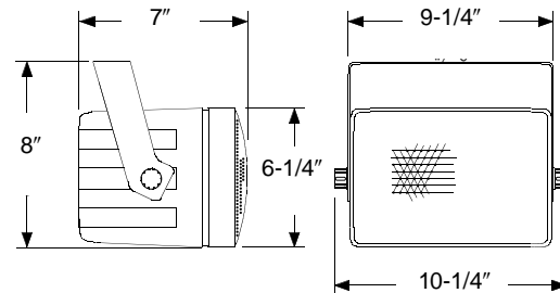
AXCA537B
